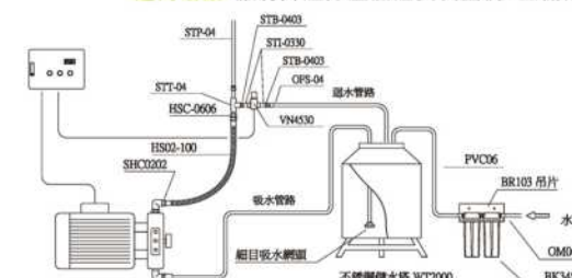
定向噴頭 廠房降溫除塵加溼安裝圖例-主機部分
