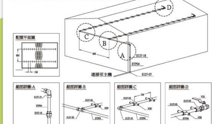
定向噴頭 廠房降溫除塵加溼安裝圖例-管路部分
